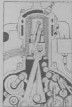
Detalle que representa el mecanismo que en Fiat se ha inventado para el motor de 6 cilindros. Puede funcionar en el sentido de la marcha ó en el sentido contrario.
